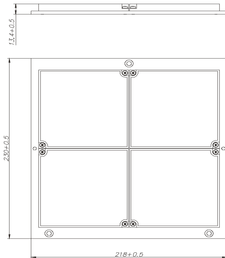
Fig. 9. Panou reflector
