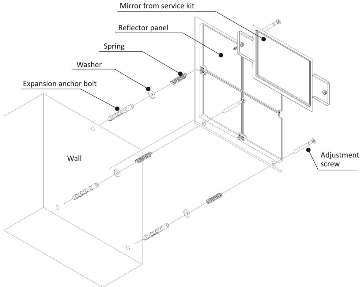
Fig. 11. Ansamblu panou reflector
