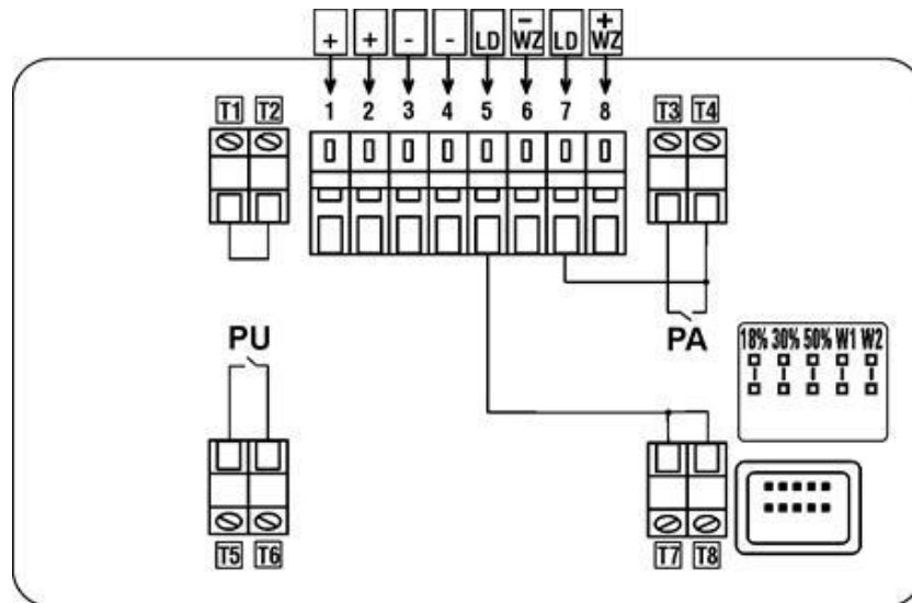
Fig. 5. Schema conexiunilor interne ale detectorului DOP-6001R și a bornelor de ieșire
