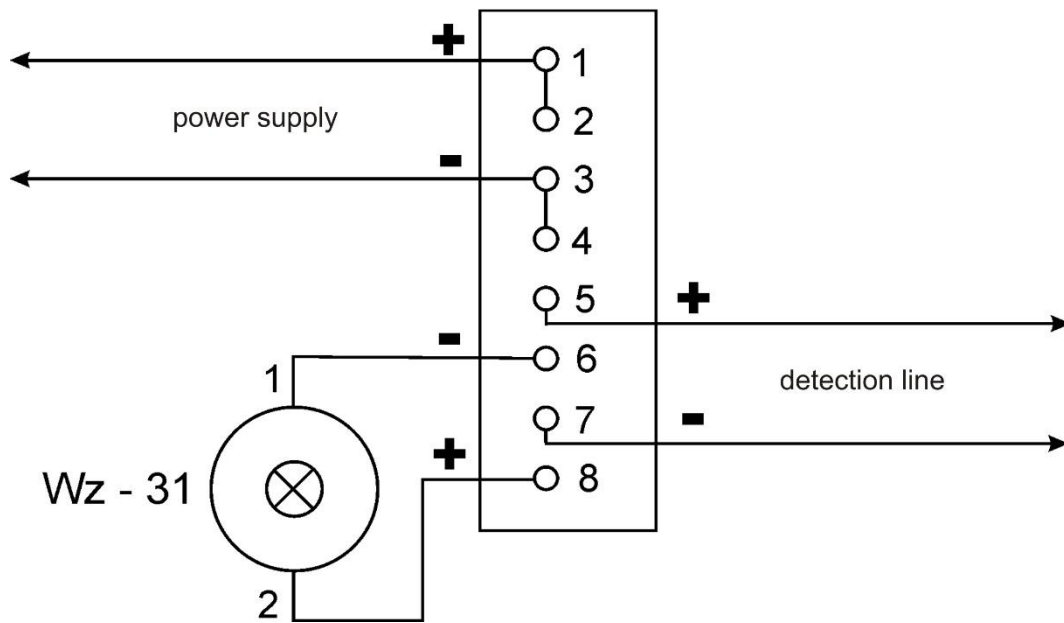
Fig. 4. Conectarea cablurilor de instalare a detectorului DOP-6001R
