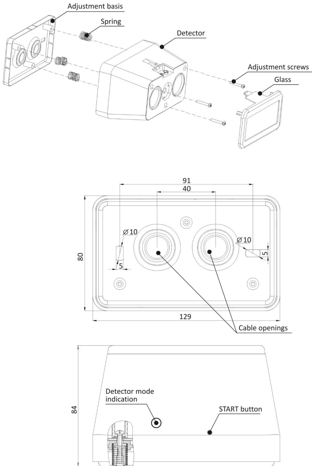
Fig. 3. Designul și dimensiunile generale ale DOP-6001R
