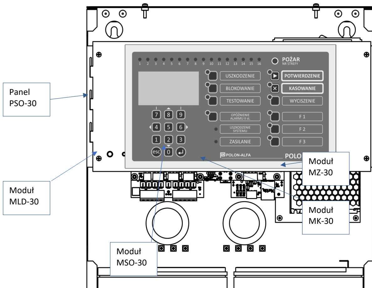
Rys. 5-2 Moduły centrali
