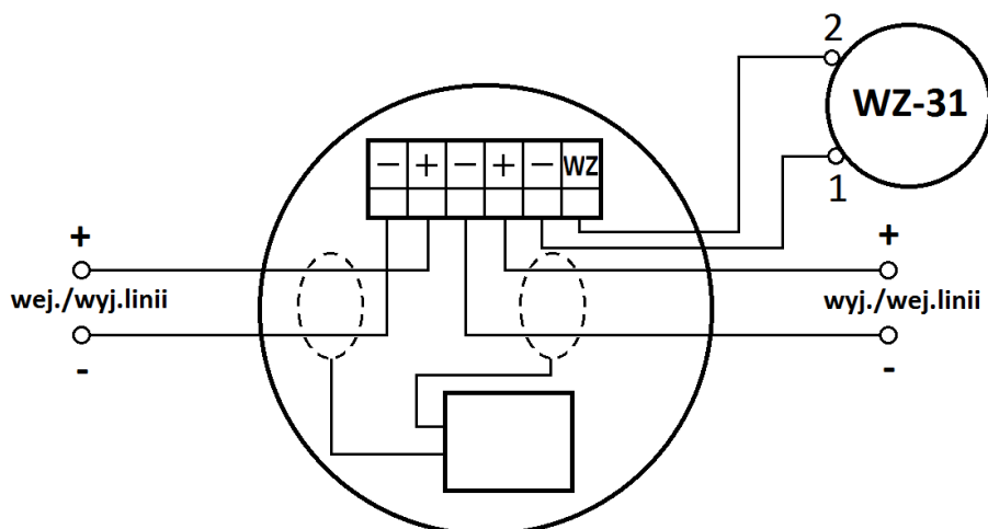
Rys.7.1 Schemat połączeń stosowany dla czujki pracującej w podstawowym trybie WZ..
