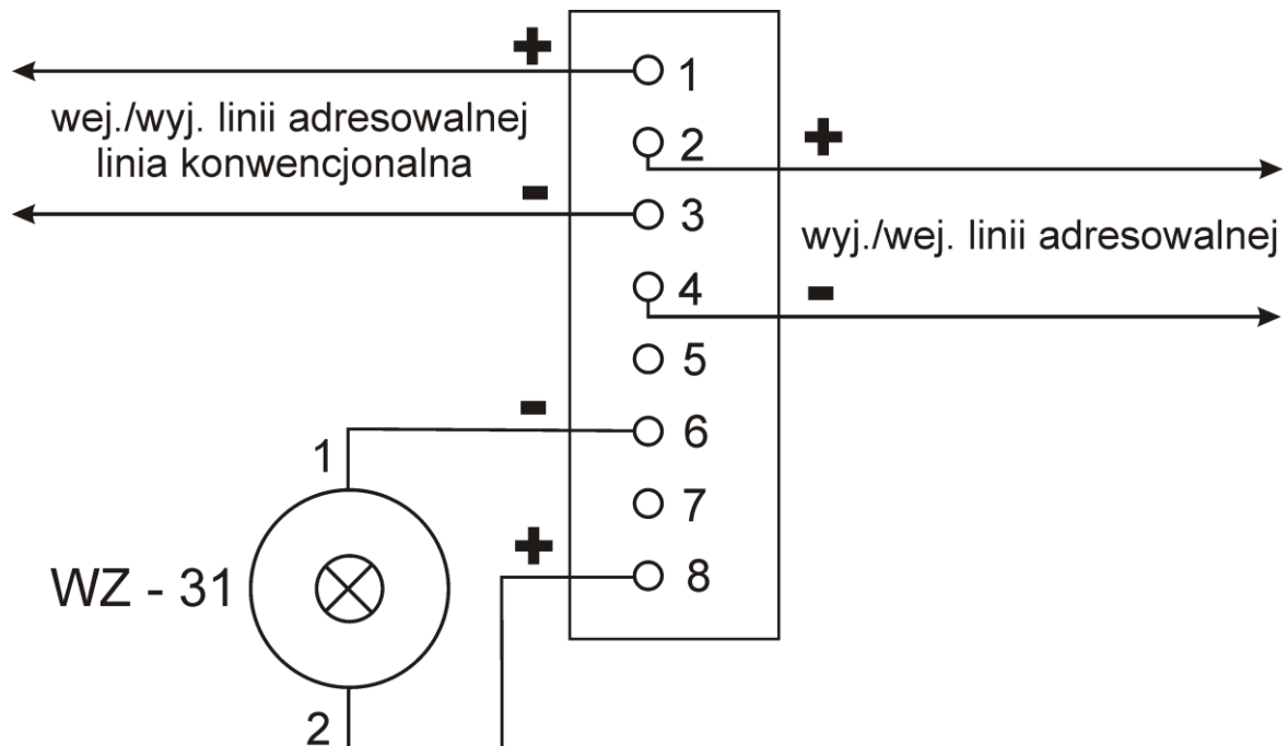
Rys 9.2. Podłączenie przewodów instalacyjnych do czujki DOP-3000
