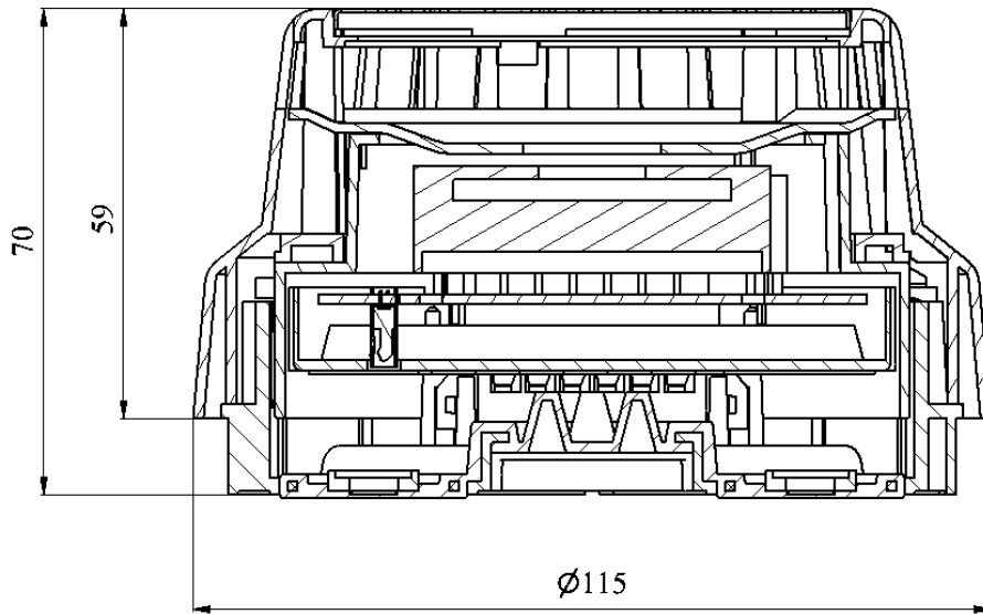
Rysunek 3/1 Konstrukcja mechaniczna sygnalizatora SAW-3000
