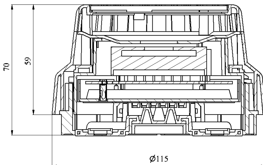
Rysunek 3/1 Konstrukcja mechaniczna sygnalizatora SAW-6100
