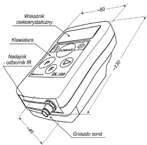
RADIOMETR RK-100-2
