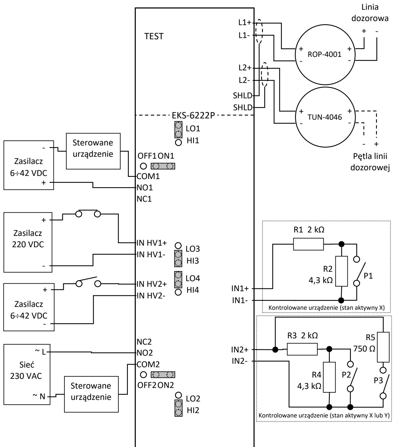
Rysunek 7-1 Przykładowy schemat połączeń EKS-6222P
