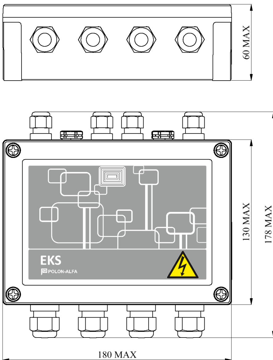
Rysunek 3-1 Wymiary EKS-6222P
