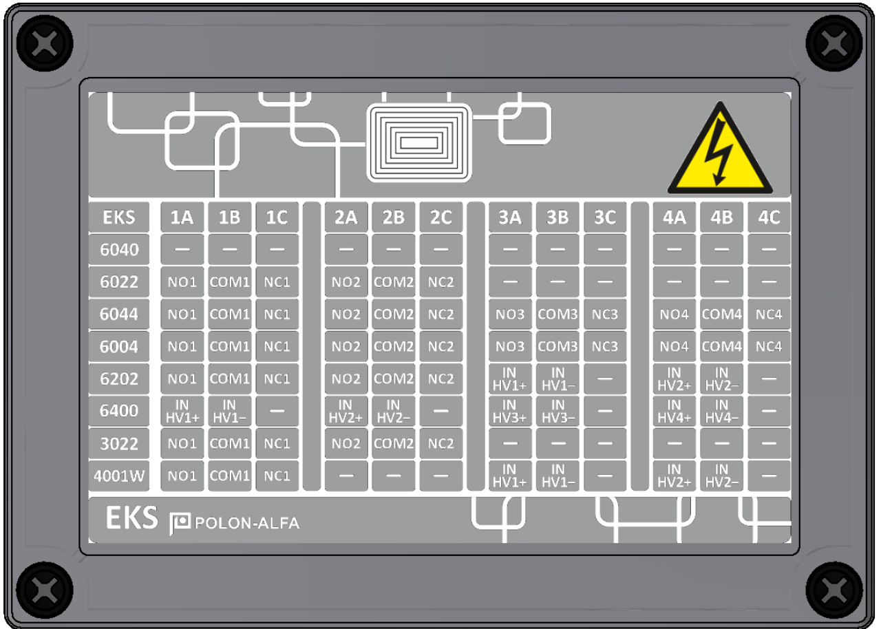
Rysunek 5 Funkcje zacisków EKS-4001W
