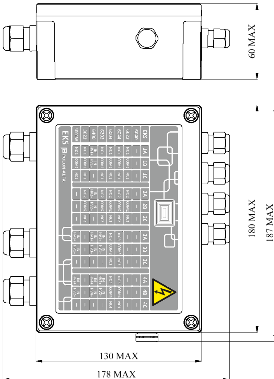
Rysunek 1 Wymiary EKS-4001W
