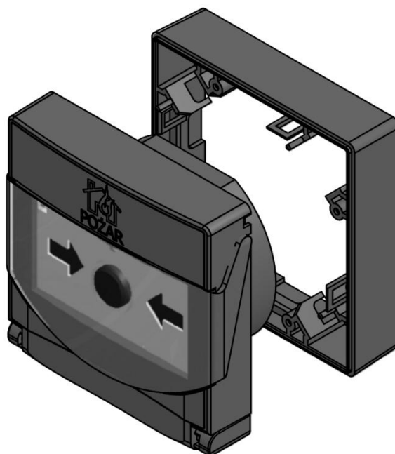
Rys. 4.1 Wygląd ogólny ręcznego ostrzegacza
