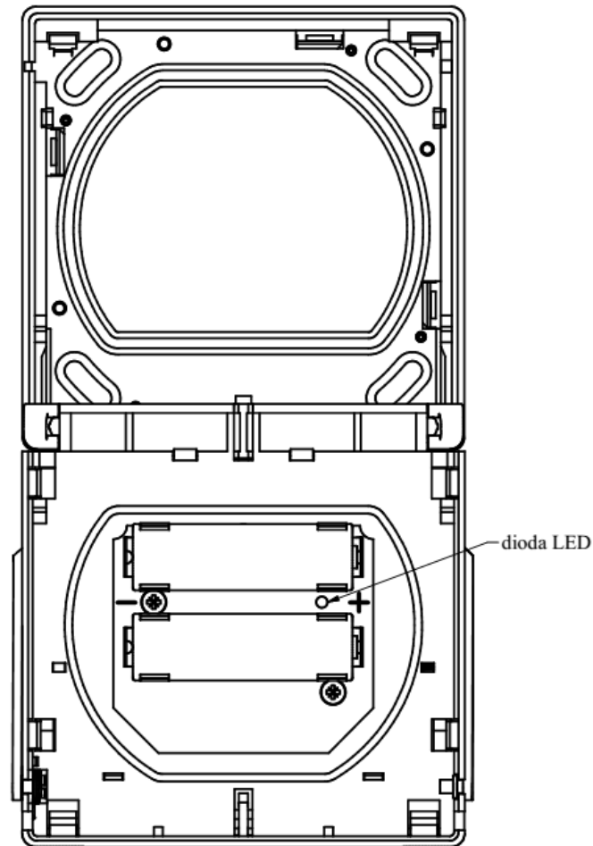
Rys. 6.2.2 Ręczny ostrzegacz po otwarciu
