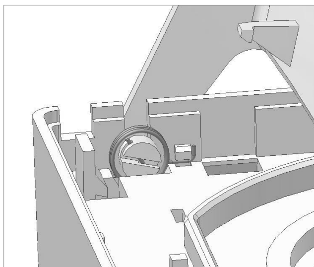
Rys. 6.3.2 Mocowanie sprężyny do korpusu
