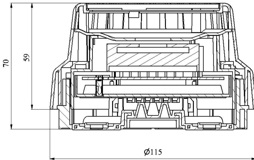
Rysunek 3/1 Konstrukcja mechaniczna sygnalizatora SAW-6000
