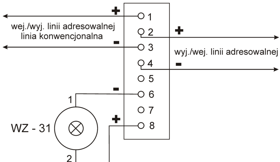
Rys 9.2. Podłączenie przewodów instalacyjnych do czujki DOP-6001
