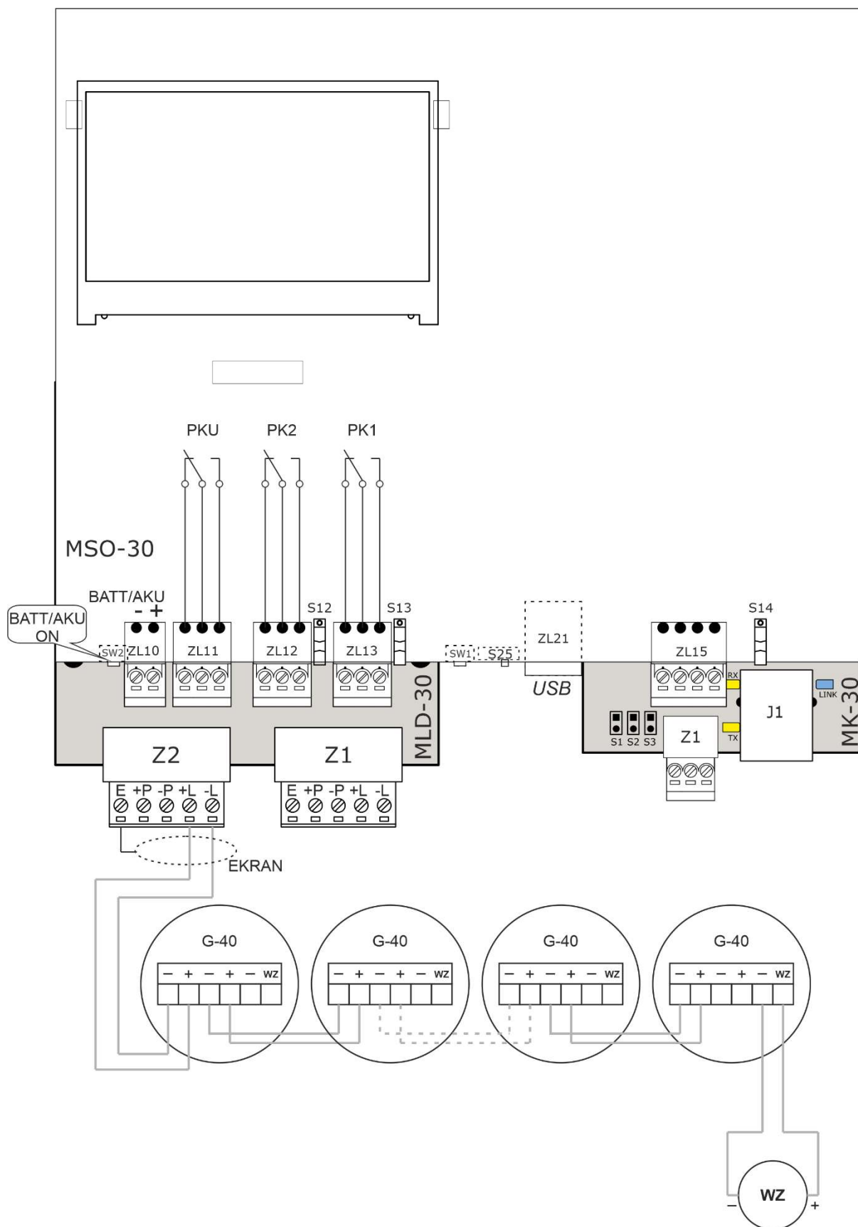
Rys. 5-9 Schemat podłączenia linii dozоровej promieniowej do modułu MLD-30
