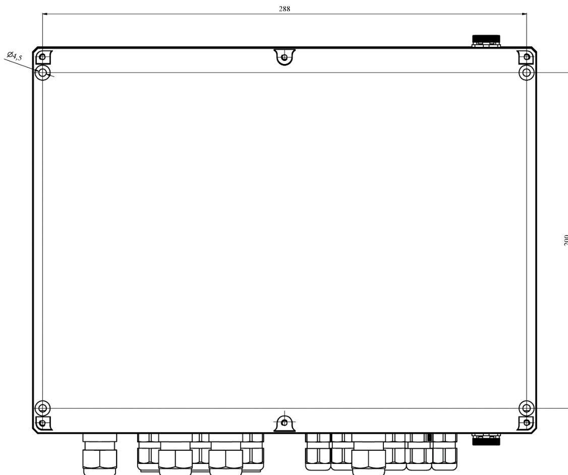
Rysunek 7.1/1. Mocowanie centrali CDG 6000-99
