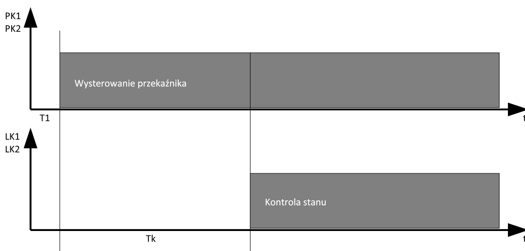
Rysunek 6.1.2/1 Kontrola zadziałania wyjść PK1 i PK2
