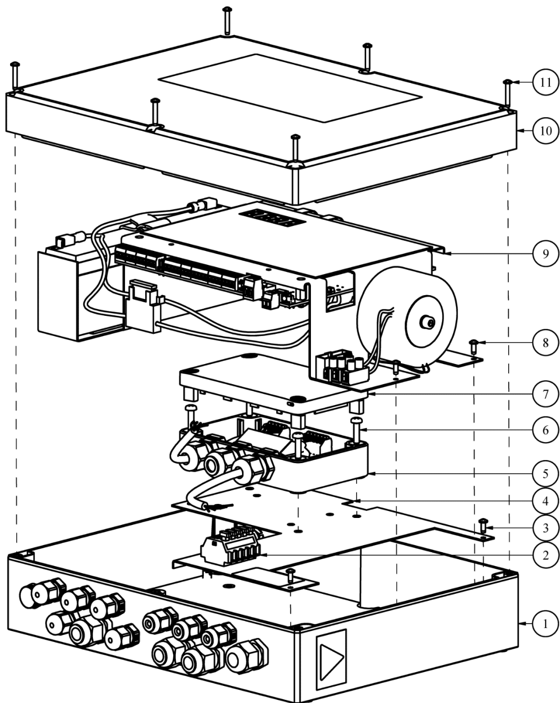
Rysunek 10.1/1 Schemat montażu AKC-6000 w centrali detekcji gazów CDG 6000-99
