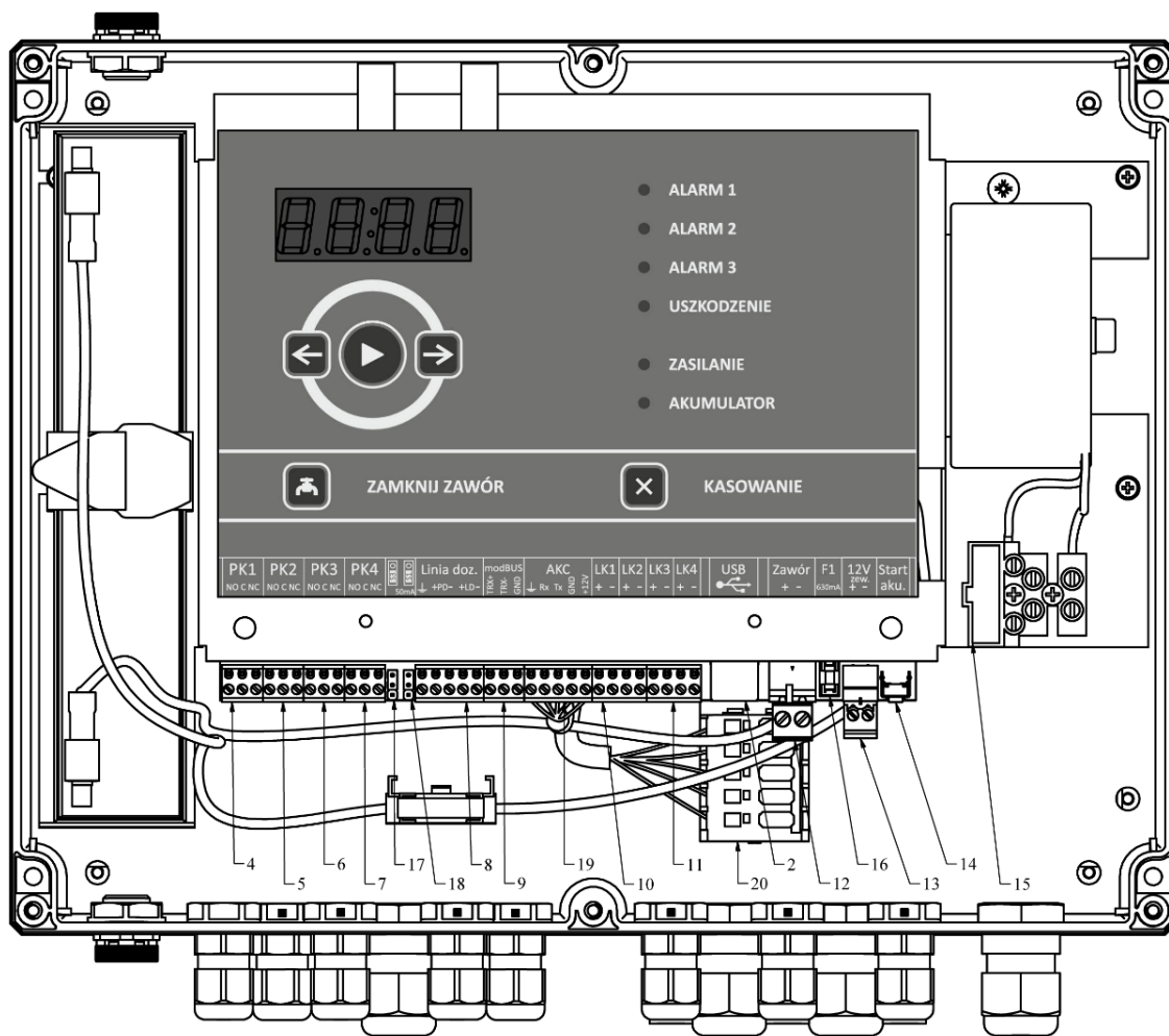
Rysunek 2.1/2. Centrala CDG 6000-99
