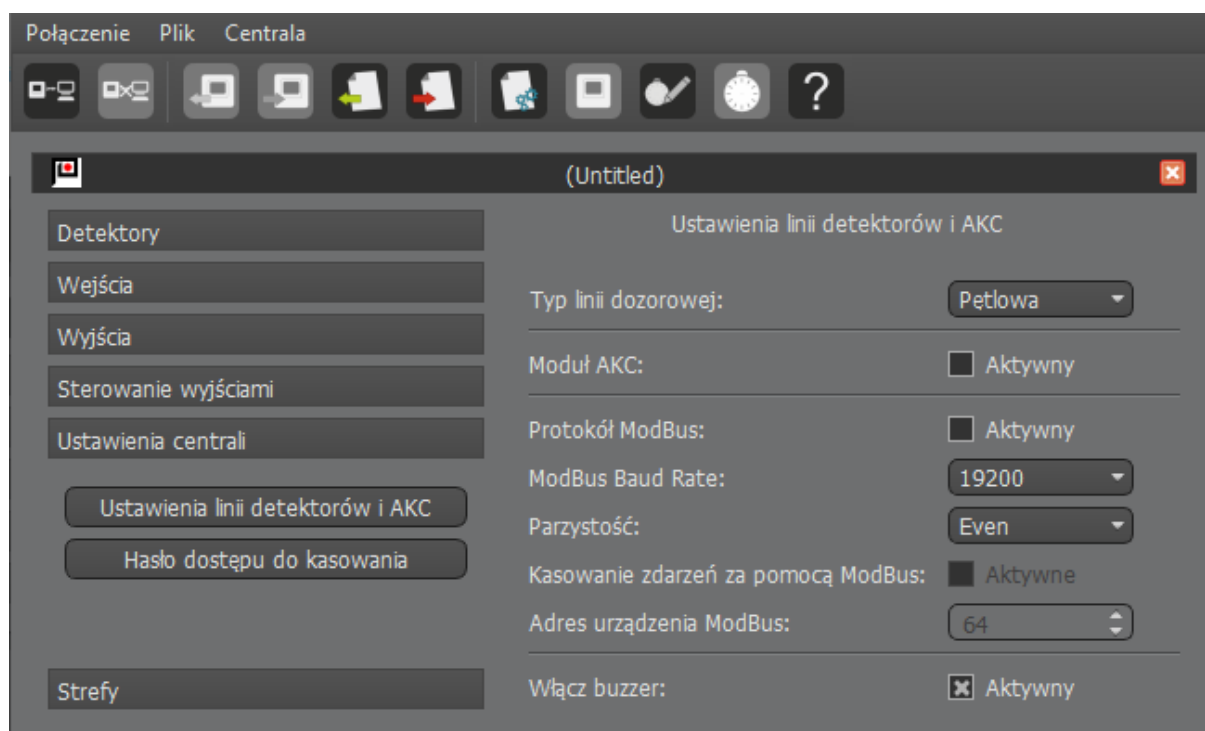
Rysunek 6.5/1 Widok zakładki konfiguratora z ustawieniami protokołu Modbus, linii oraz AKC
